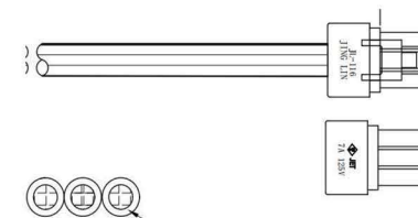
3P連続線（オスとメスソケット） (7A・125V)
